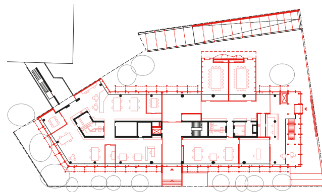
Grundriss Erdgeschoss
