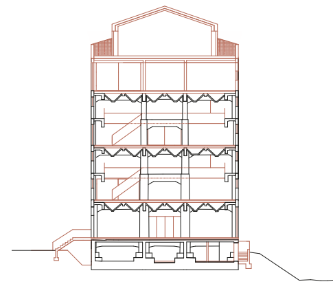
Schnitt B-B
