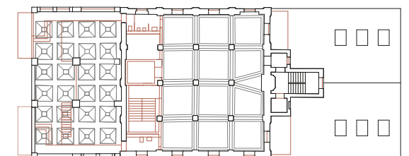
Grundriss 2. Obergeschoss mit Galerieebene
