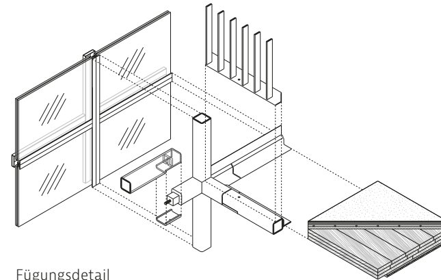
Fügedetail der Hybridbauweise Holz, Stahl, Glas
