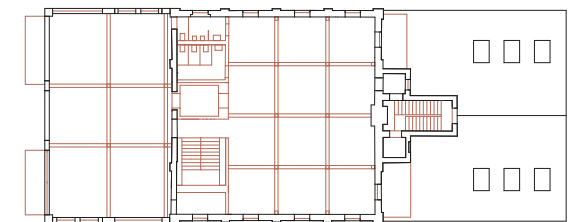
Grundriss 5. Obergeschoss mit neuen Stützen
