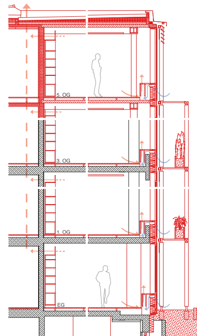
Fassadenschnitt
