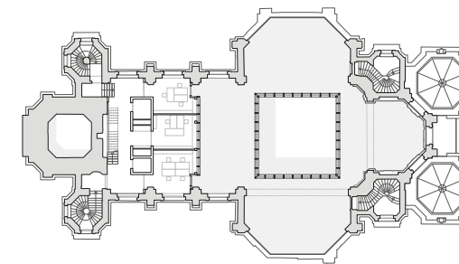
Grundriss 1. Obergeschoss
